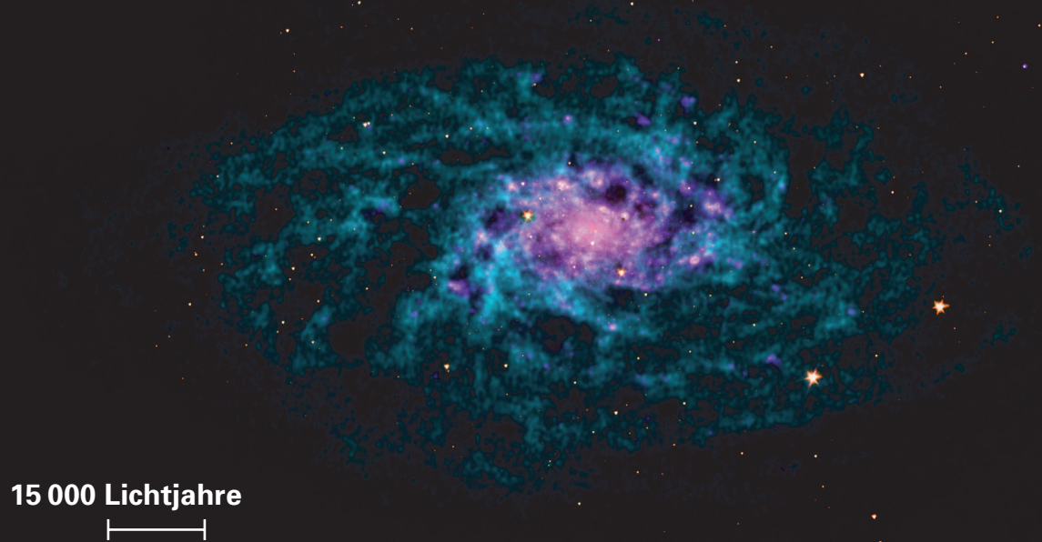
NGC 2403 – Gas und Sterne
