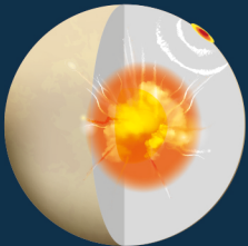
Doppeldetonnations-SN-Ia
